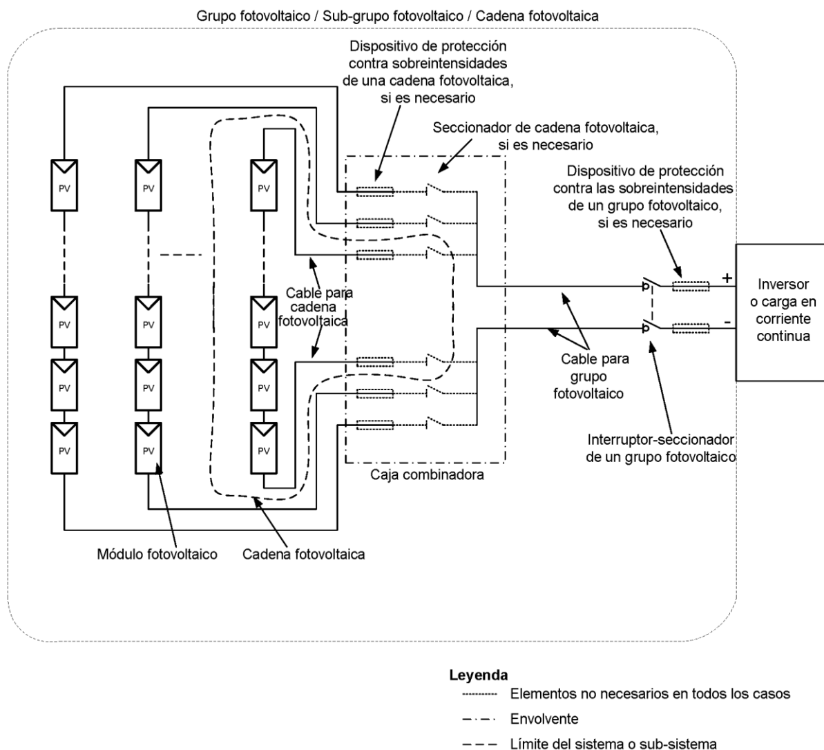
Figura 712.A.1 – Grupo fotovoltaico de una sola cadena o múltiples cadenas conectadas en paralelo
